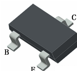
SOT- 23
