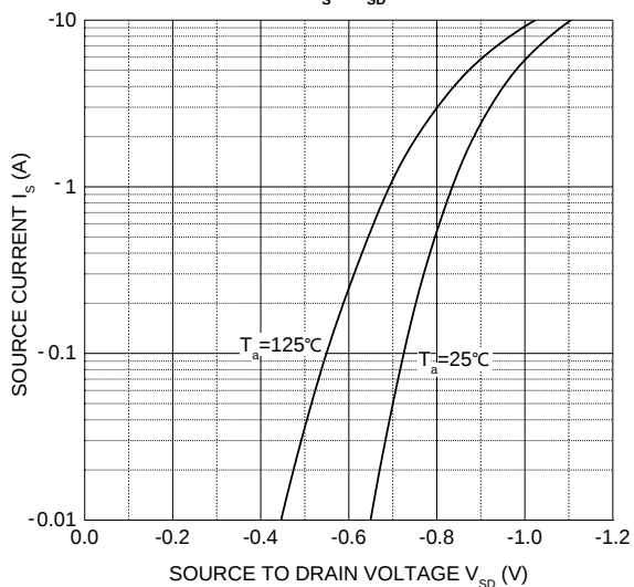
I_S - V_{SD}
