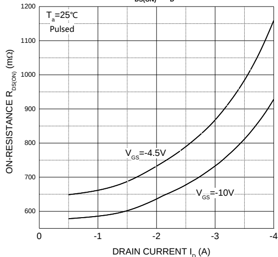
R_{DS(ON)} - I_D
